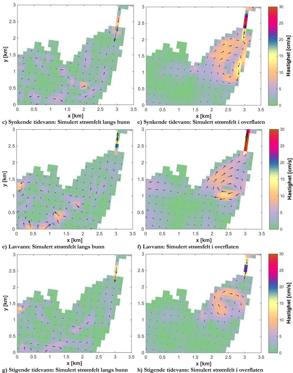
Figur 28. Simulert strømfelt for 1. mai 2014. Simuleringene er utført med en kurvelineær 3D modell i ROMS. Simuleringene er utført av MET.
